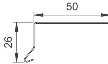
Murkrone type 10Z og 10ALU - Standard
