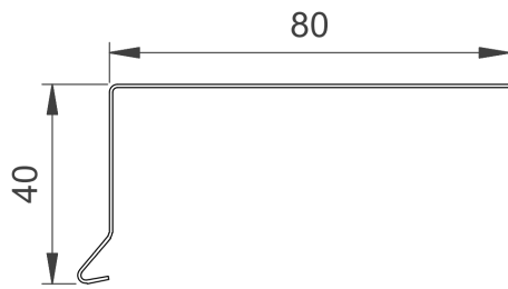
Murkrone type 10, 10S og 10A – Standard
