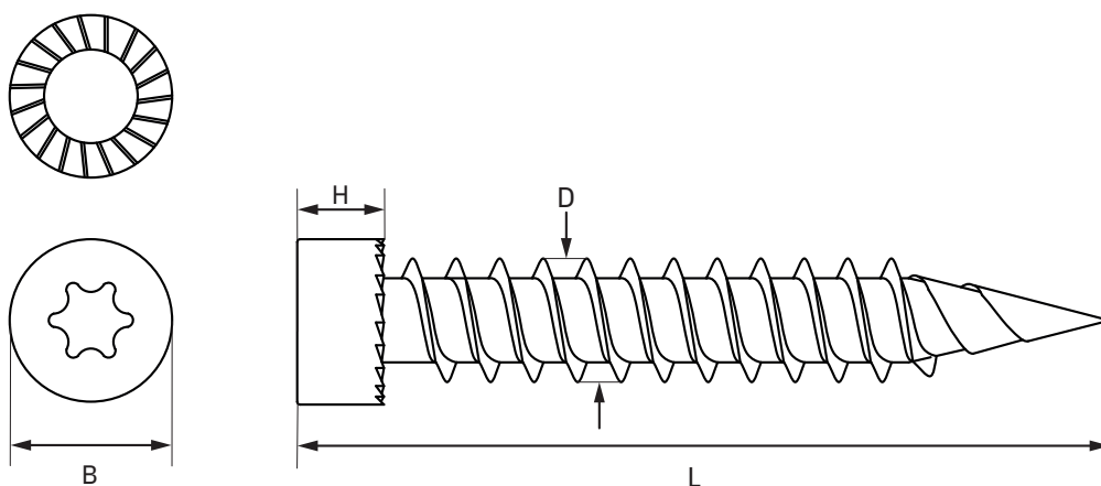
Tegning af DANOloft skrue til visualisering af mål i tabellen Produktdata
