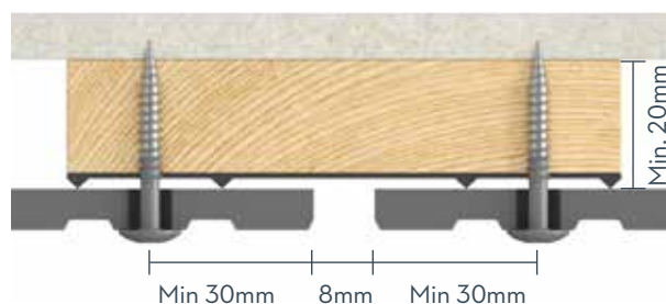
Figur 1. Cembrit Patina Inline installation på bagvedliggende forskalling.
