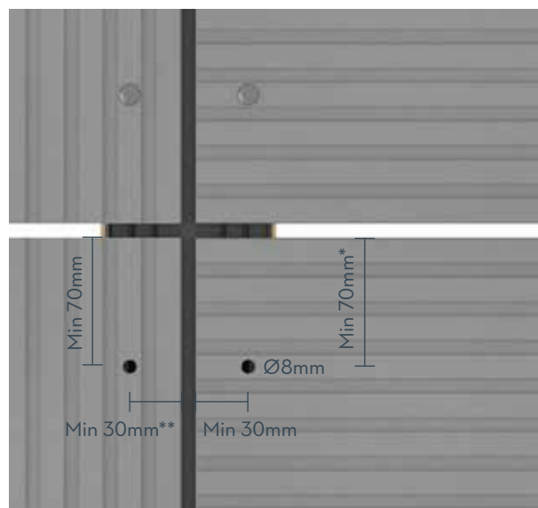
Figur 3. Cembrit Patina kantafstande.
