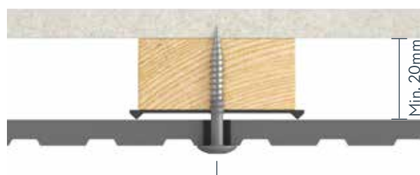
Figur 2. Montering af Cembrit Patina Inline på bagvedliggende forskalling.
