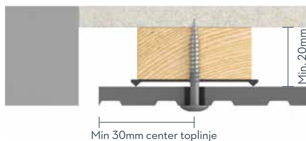
Figur 4. Skruelacering på tildannede plader ifm. Cembrit Patina Inline.
