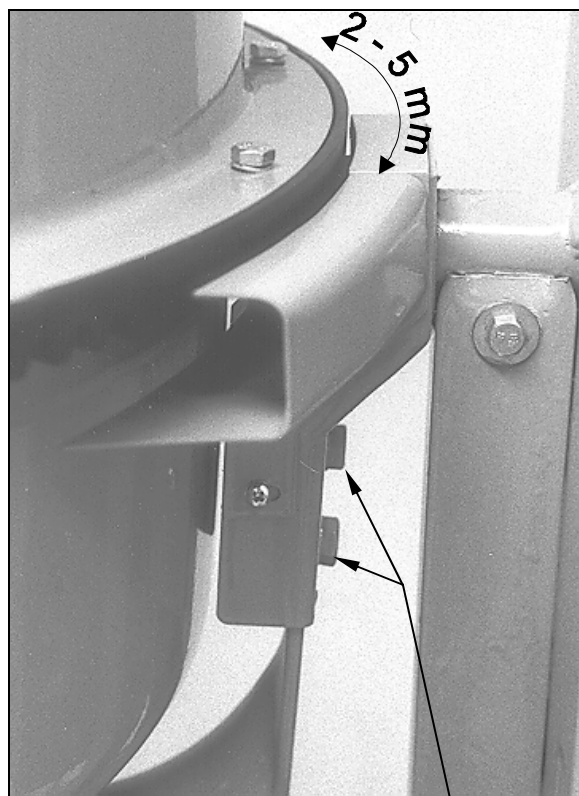
M10x25
