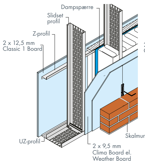
Eks. 1: Ydervæg med skalmur
