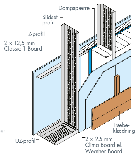
Eks. 2: Ydervæg med let beklædning
