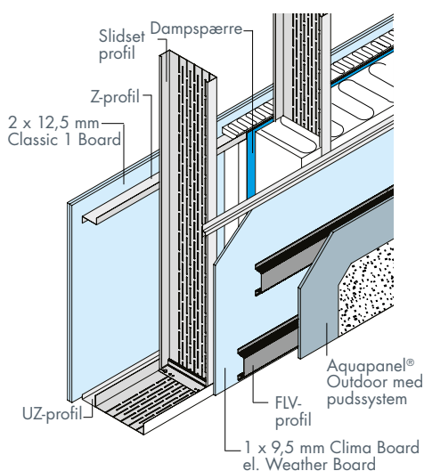
Eks. 3: Ydervæg med Aquapanel® og pudssystem
