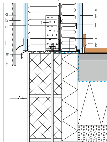
YB12: Fundamenttilslutning
