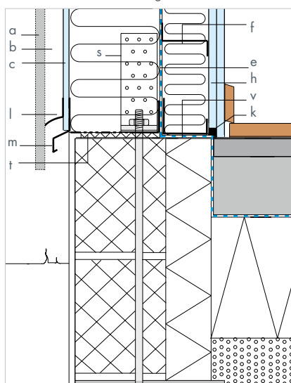
YU10: Fundamenttilslutning
