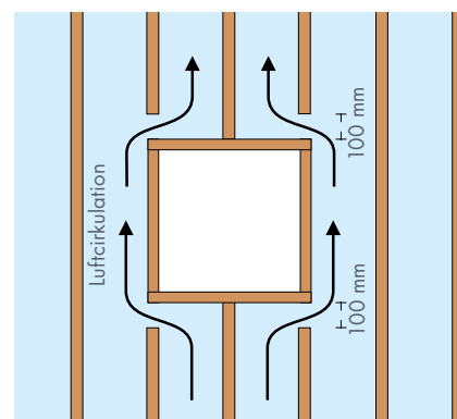
Placering af afstandslister omkring vindue.
