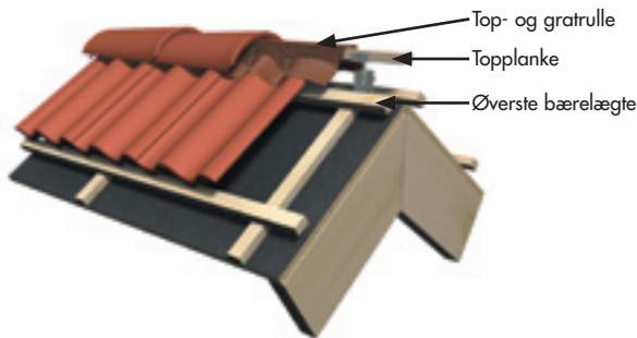
Figur 4. Afstanden fra topplankens centrum til øverste bærelægte skal være ca. 40 mm, se tabel 3. Afprøv at rygningstenen overlapper øverste række tagsten på forsvarlig vis.
