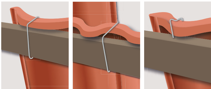
Figur 12a. Nakkeclips til fastgørelse af 1K og 2K tagsten og specialsten. Det anbefales at fastgøre alle sten i øverste og nederste række, og alle sten ved udhæng mv.
