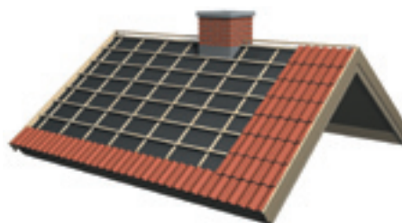
Figur 10. Læg nederste række fra højre mod venstre. Læg en hel række op i højre side til rygningen. Sørg for at stenene ligger i vinkel. Når du har oplagt 2-3 rækker, kontrolleres om taget er i vinkel.
