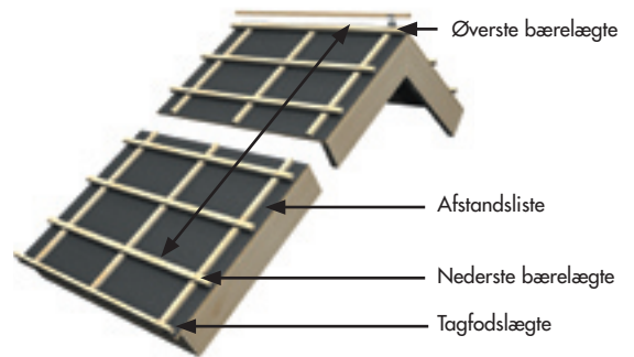
Figur 5. Udregn antallet af tagsten. Se også tabel 5.
