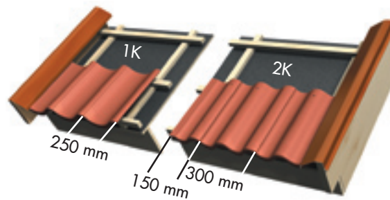
Figur 9. Opdel tagbredden i antal tagsten. Husk at den sidste sten ud mod ventre gavl dækker 330 mm for 2K og 280 mm for 1K.
