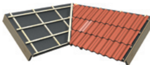
Figur 16. Ved skotrender anvendes halvsten (findes kun til 2K) for at undgå meget små stykker sten. Halvstenene er markeret på billedet.
