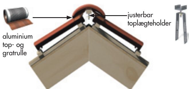
Figur 13. Anvendelse af Benders aluminium top- og gratrulle. Let at montere, skal blot ruller ud over toplægten, og lægges ned over de øverste rækker tagsten, hvorefter beskyttelsespapiret fjernes og rullen presses ned i tagstenens bølger.
