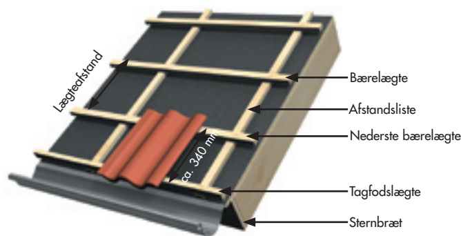
Figur 2. Lægteafstand måles fra overkant til overkant. Vær opmærksom på, at der fra tagfodslægtens nederste kant til nederste bærelægtes overkant ikke må være mere end 340 mm. Husk også på, at tagfodslægten skal være 20 mm højere end de øvrige bærelægter, da den nederste række tagsten ikke hviler på andre tagsten. Højdeforskellen kan udlignes ved brug af fuglegitter med ventilation.
