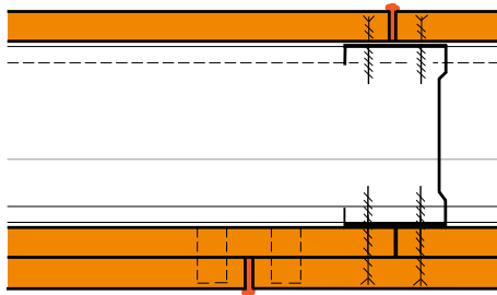
Klæbefugesamling.
