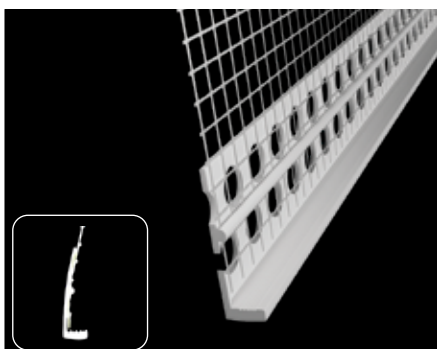
LIP Bundliste Varenr.: 33021 Dim.: 6 mm x 100 mm x 2 m.
