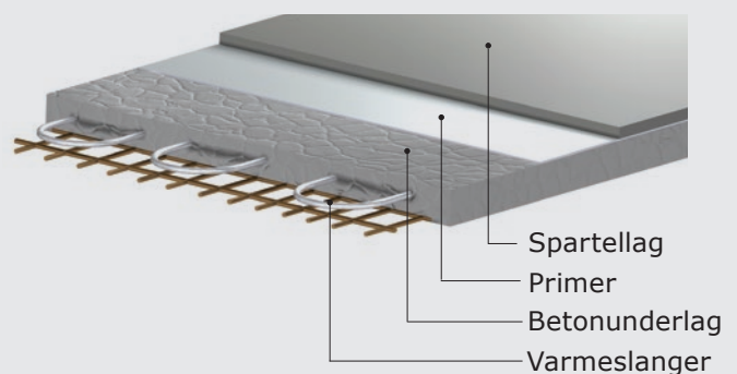
Spartling på betonunderlag med vandbårne varmeslanger
