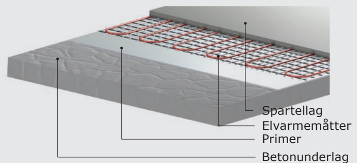
Spartling på betonunderlag med elvarmemåtter/kabler
