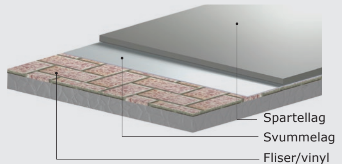
Spartling på eksisterende fliser/vinyl
