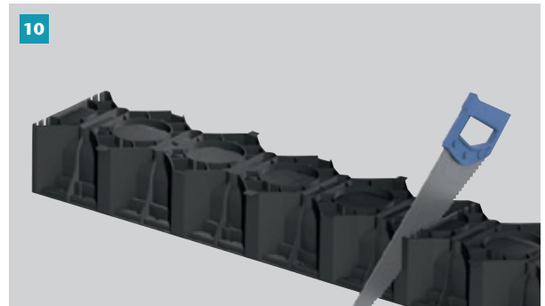
Selve drænet kan afkortes til en vilkårlig længde. OBS! Skal den afkortede ende tilsluttes endnu et dræn eller hjørnestykke, skal drænet afkortes ved 50 cm, hvor der er markeret en skærelinie.
