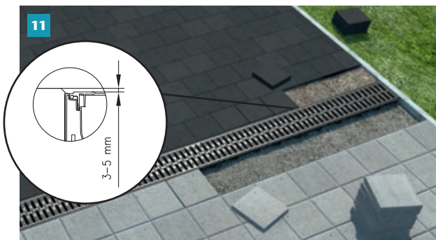
For fastholdelse lægges tilstødende belægningssten i beton. Bemærk overkant af belægningssten skal være 3-5 mm over ristens overkant.
