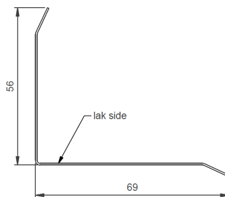
Facadeinddækningsprofil type 2 – standard
