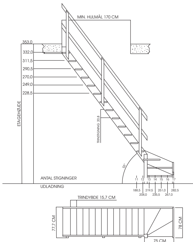
Normandie kvartsvingstrappe
