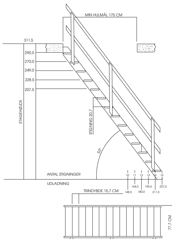
Normandie ligeløbstrappe
