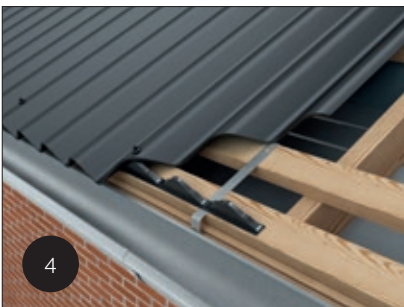
4 Ventilation ved tagfod kan etableres ved montering af Swisspearl Plastudhængsklodser med ventilation. Se side 17.
