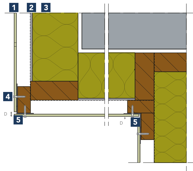
Detailskitse 1-201
