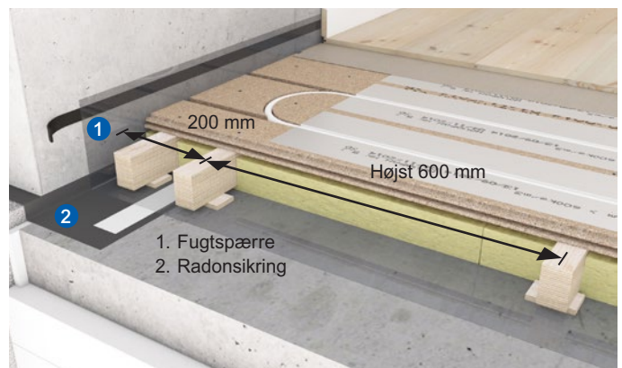
Figur 2 Klimagulv lagt på strøer med fræsedespor udført på byggepladsen.
