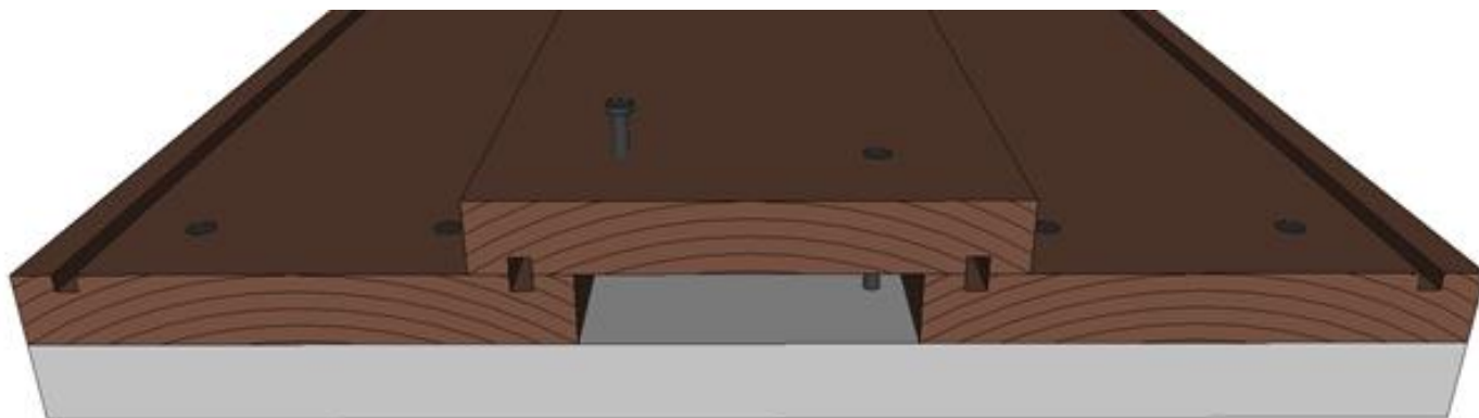
Figur 2 Montering af rektangulære tagbrædder
