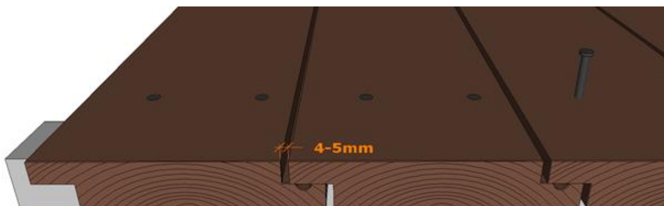
Figur 1 Montering af dobbeltfalsede tagbrædder
