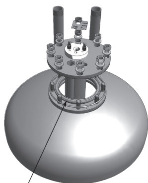
Pakning Figur 9
